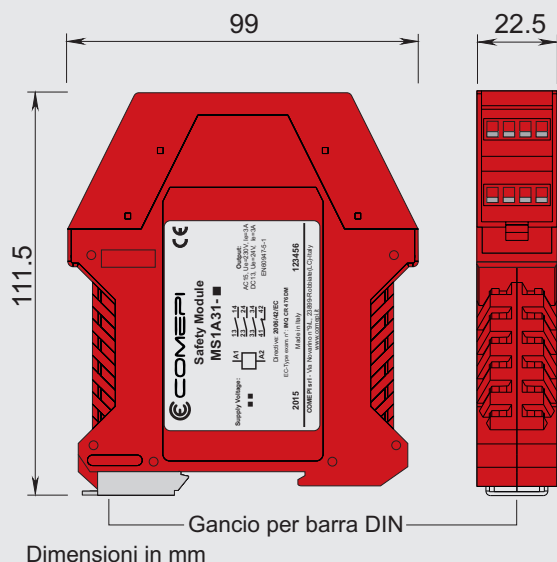
Fig.1.1 - Dimensioni meccaniche
